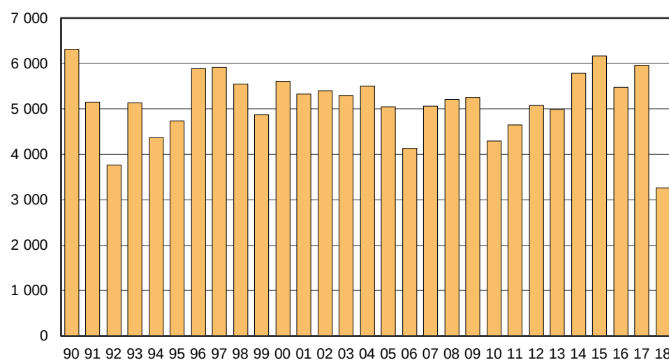
Figur A. Spannmål. Totalskördar 1990–2018
