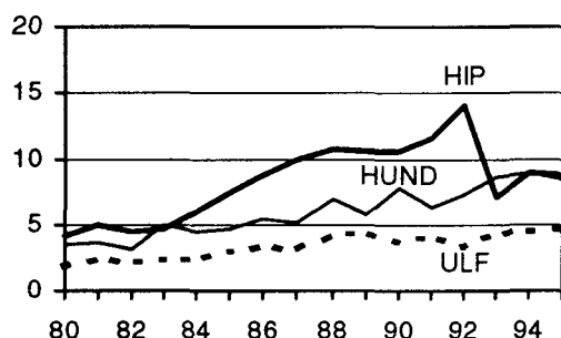
Diagram 3. Andel ej anträffade 1980-1995 för HIP, HUND och ULF. Ovägt årsgenomsnitt i procent.
