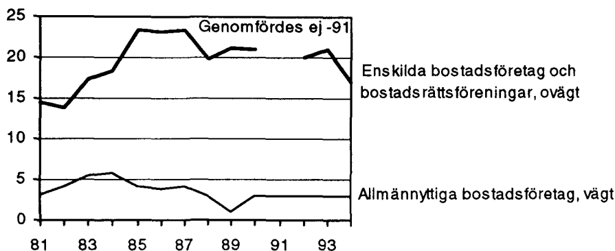
Diagram 8. Bortfallsutvecklingen för IKU 1981-1994.
