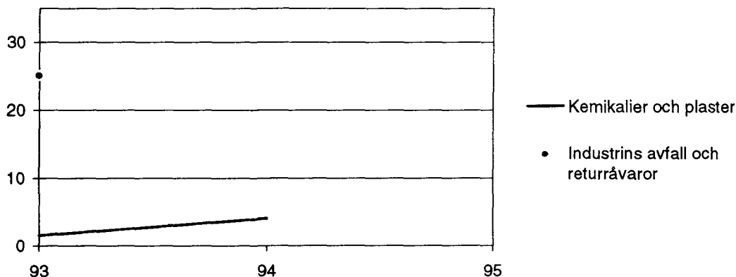
Diagram 6 Bortfallsutvecklingen för Industrins avfall och returråvaror samt Kemikalier och plaster
