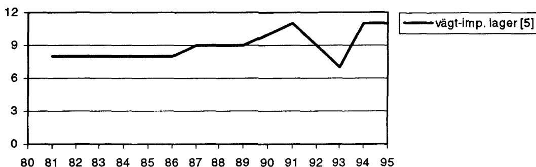
Diagram 6. Bortfallet i Lagertypstatistiken 1981-1995, procent.
