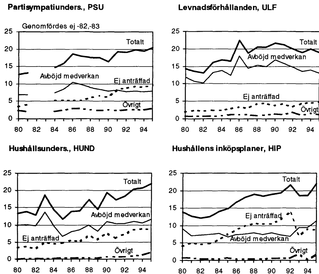
Diagram 2. Bortfallsutvecklingen i PSU, ULF, HUND och HIP 1980-1995. Övägt årsgenomsnitt i procent.
