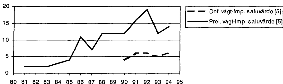
Diagram 3. Bortfallet i Industristatistiken 1981-1995, procent
