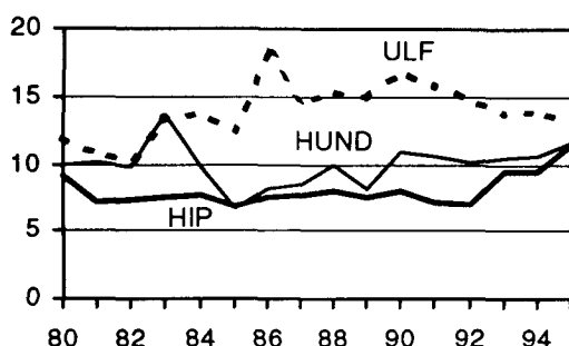
Diagram 5. Andel avböjd medverkan 1980-1995 för HIP, HUND och ULF. Ovägt årsgenomsnitt i procent.
