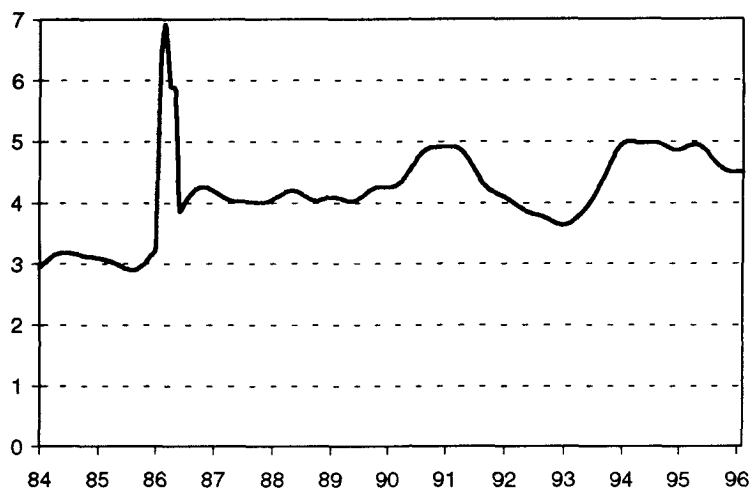
Diagram 1 Trendcykel-kurva för andel som avböjt medverkan i nya paneler i AKU.
