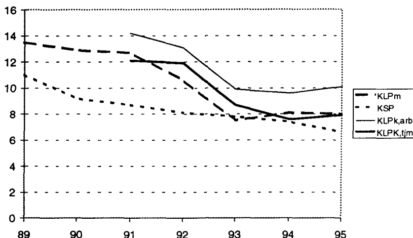
Diagram 4 Bortfall i kortperiodiska undersökningar 1989-1995. Ovägt [1]. Årsgenomsnitt. Procent.
