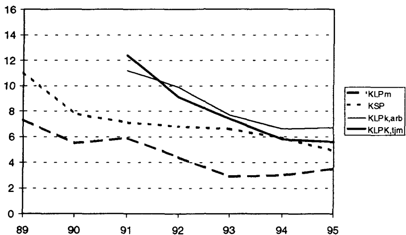
Diagram 5 Bortfall i kortperiodiska undersökningar 1989-1995. Storleksvägt [4] med antal anställda enligt CFAR. Årsgenomsnitt. Procent.
