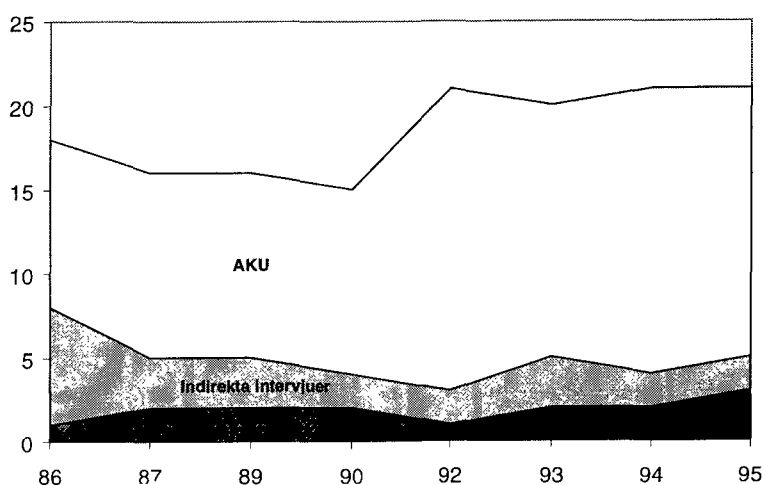
Diagram 2 Bortfallet i personalutbildningsstatistiken 1986-1995. (Obs! Ingen undersökning 1988 och 1991)
