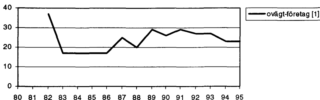
Diagram 8. Bortfallet i Omsättningsstatistiken 1982-1995, procent.
