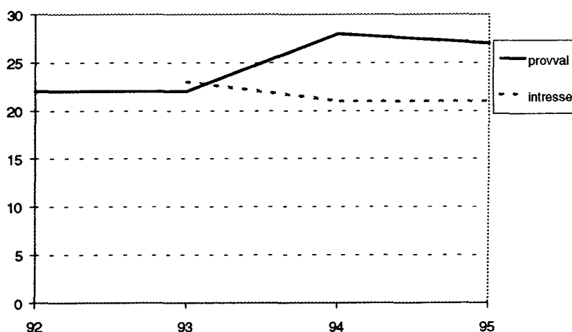
Diagram 3 Bortfall i Provval till gymnasieskolan. Ovägt [1]. 1992-1995. Bortfall i Gymnasieungdomars intresse för högre studier . Ovägt [1].1993-1995
