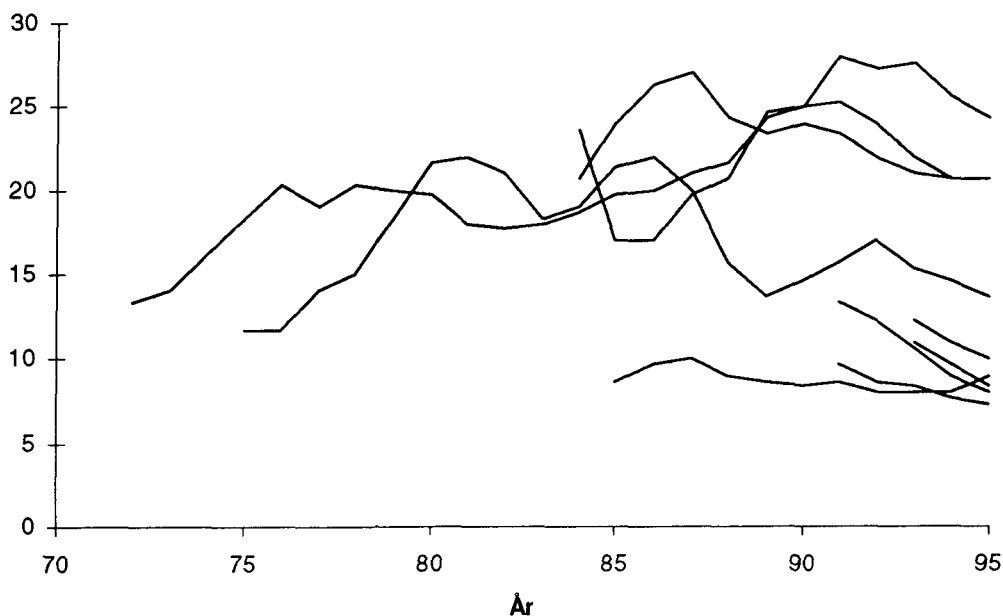
Figur 1. Ovägt bortfall för företagsundersökningar. Utjämnade serier.
