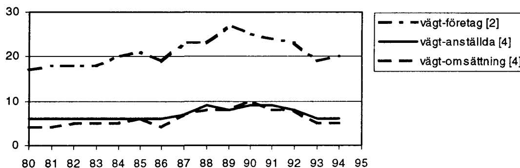
Diagram1. Bortfallet i Finansstatistiken 1980-1995, procent.
