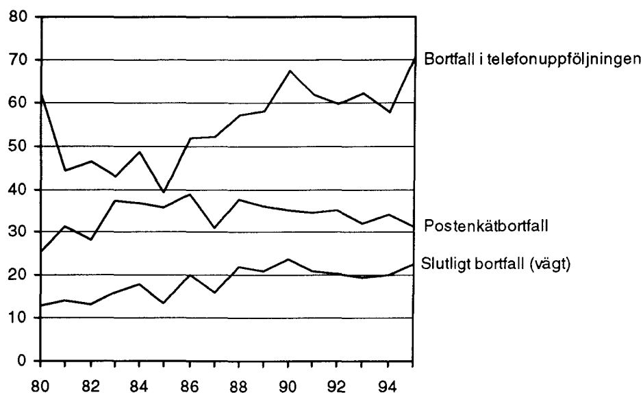
Diagram 7. Bortfallsutvecklingen i omnibusundersökningarna 1980-1995. Årsgenomsnitt i procent.
