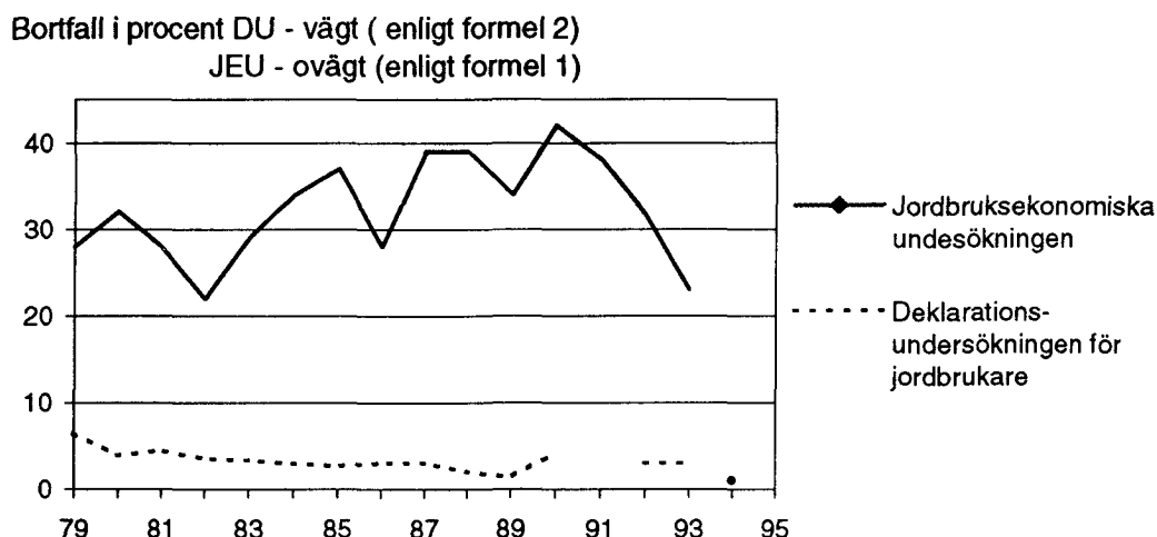
Diagram 3 Bortfallsutvecklingen för Jordbruksekonomiska undersökningen (JEU) och Deklarationsundersökningen för jordbrukare (DU)
