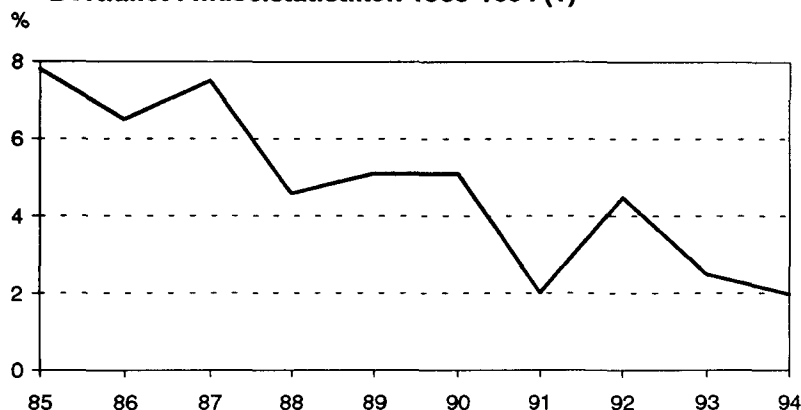
Diagram 1. Bortfallet i museistatistiken 1985-1994 (1) 1
