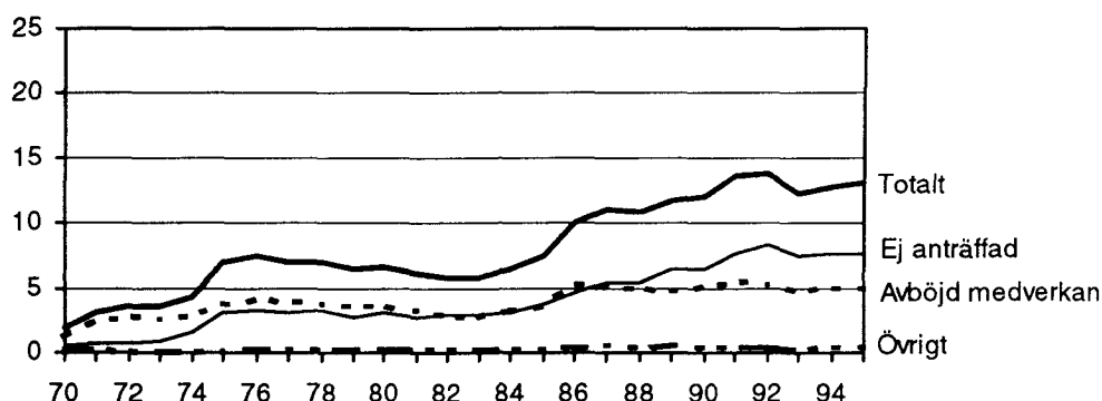
Diagram 1. Bortfallsutvecklingen i AKU 1970-1995. Övägt årsgenomsnitt i procent.
