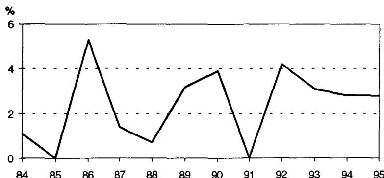
Diagram 4 Bortfallet i kreditmarknadsstatistiken (1) 1
