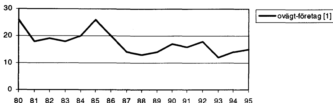
Diagram 4. Bortfallet i Investeringsenkäterna 1980-1995, procent
