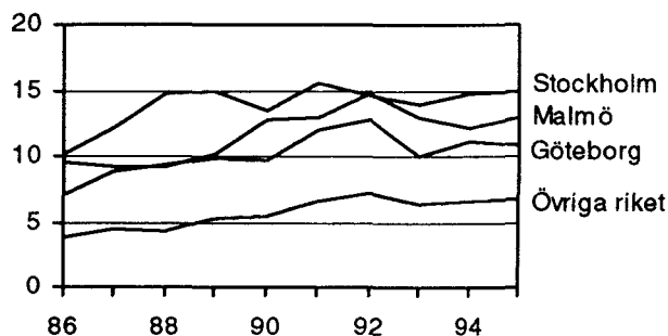
Diagram 4. Regional uppdelning av de ej anträffade i AKU 1986-1995. Ovägt årsgenomsnitt i procent.
