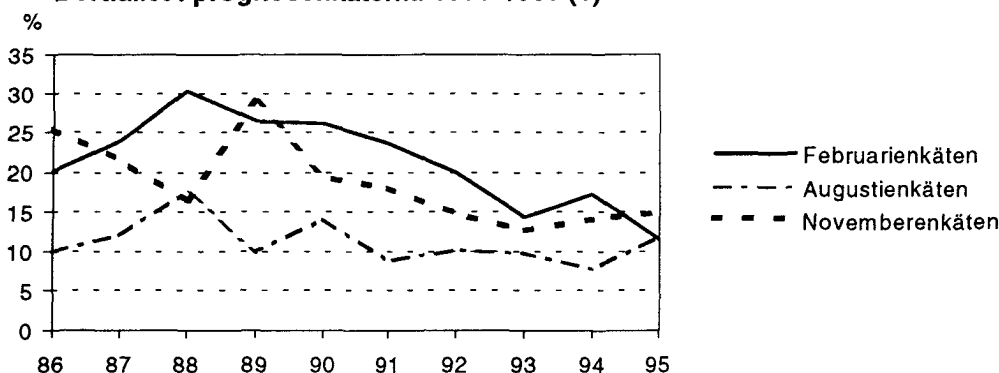
Diagram 3. Bortfallet i prognosenkäterna 1986-1995 (1) 1
