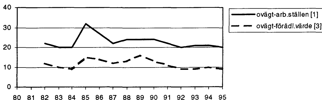
Diagram 5. Bortfallet i Kapacitetsenkäten 1982-1995, procent.
