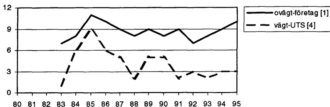
Diagram 2. Bortfallet i FUTS:en 1983-1995, procent
