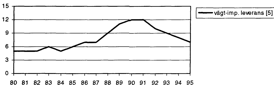
Diagram 7. Bortfallet i Leverans- och orderstatistiken 1980-1995, procent.
