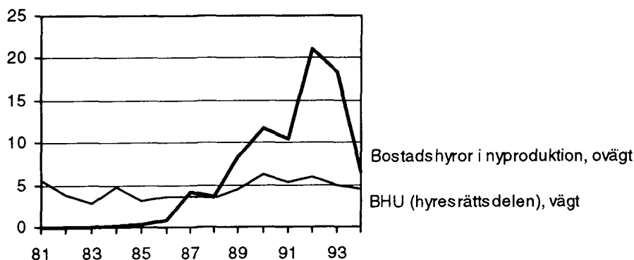
Diagram 9. Bortfallsutvecklingen för Bostadshyror i nyproduktion samt för BHU (hyresrättslägenheter) 1981-1994.
