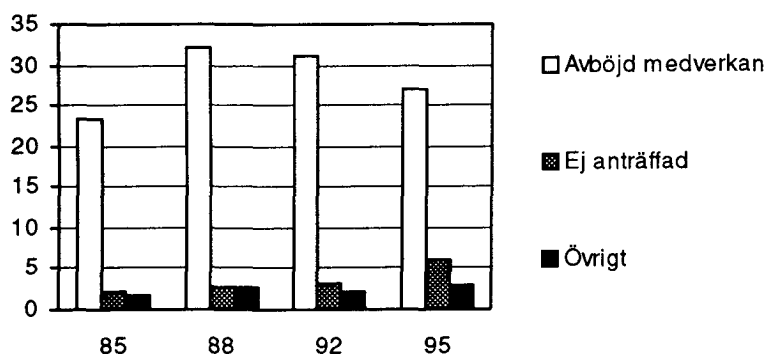
Diagram 6. Bortfallsutvecklingen i HUT/Utgiftsbarometern 1985, 1988, 1992 och 1995. Ovägt årsgenomsnitt i procent.
