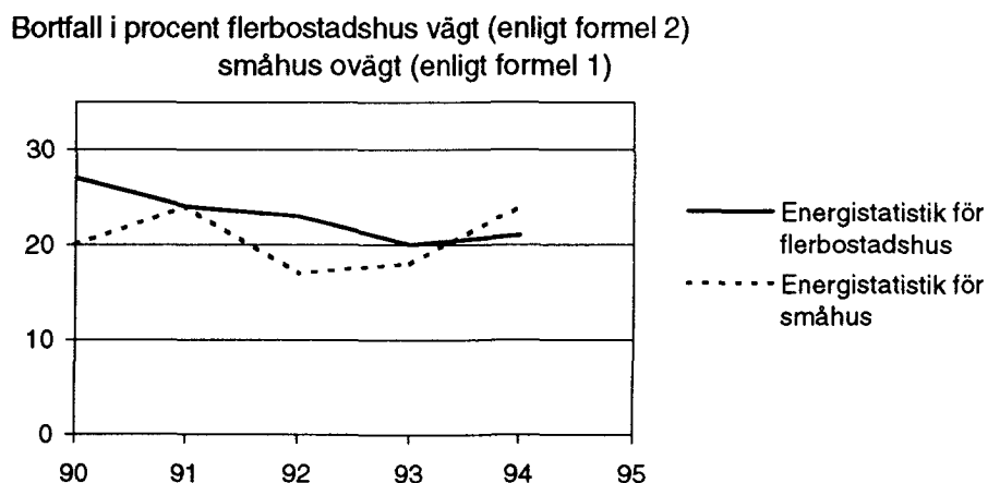
Diagram 4 Bortfallsutvecklingen för energistatistik för Småhus samt Flerbostadshus
