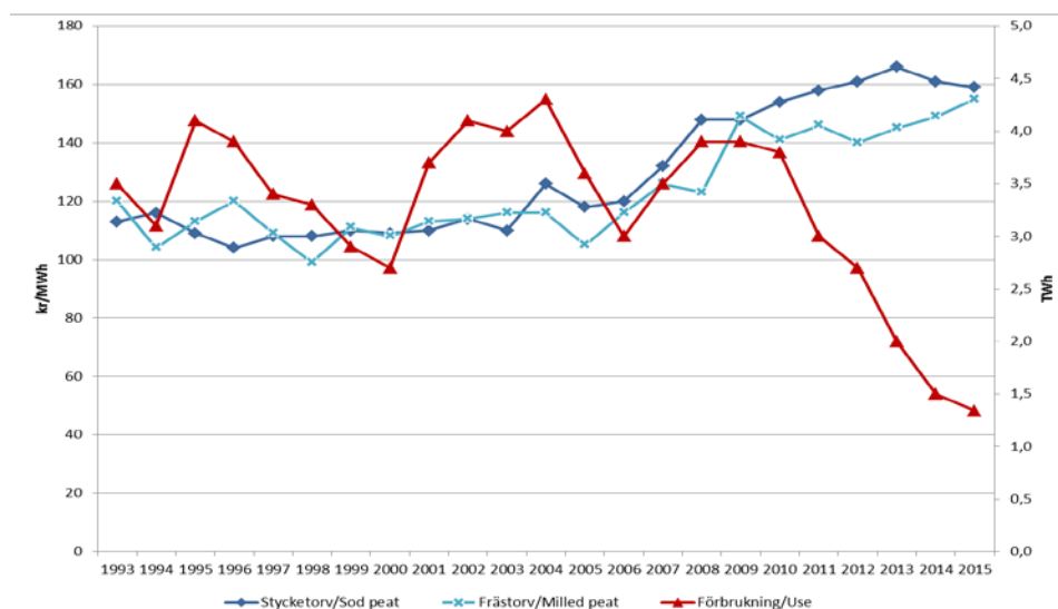
Diagram 6. Löpande priser för stycke- och frästortv (kr/MWh) samt användning av torv (TWh), 1993–2015 Nominal prices for milled peat, sod peat (SEK/MWh) and use of peat (TWh)
