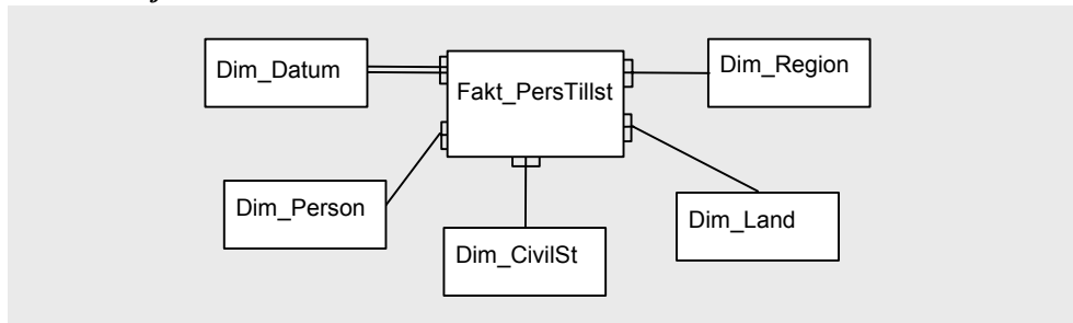
Bild 9.2 Stjärnmodell
