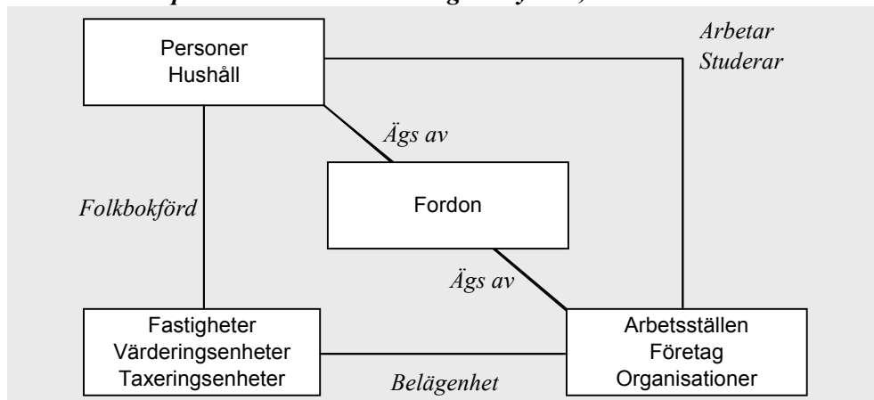
Bild 2.1 Konceptuell modell av SCB:s registersystem, version 1
